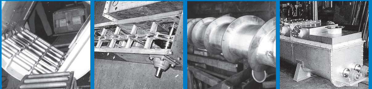
再生・改修の実績 鋳物の型枠(2tクラス)の反転機の再生/大型ショットブラストの改修/スクリーンプレスの更新等
